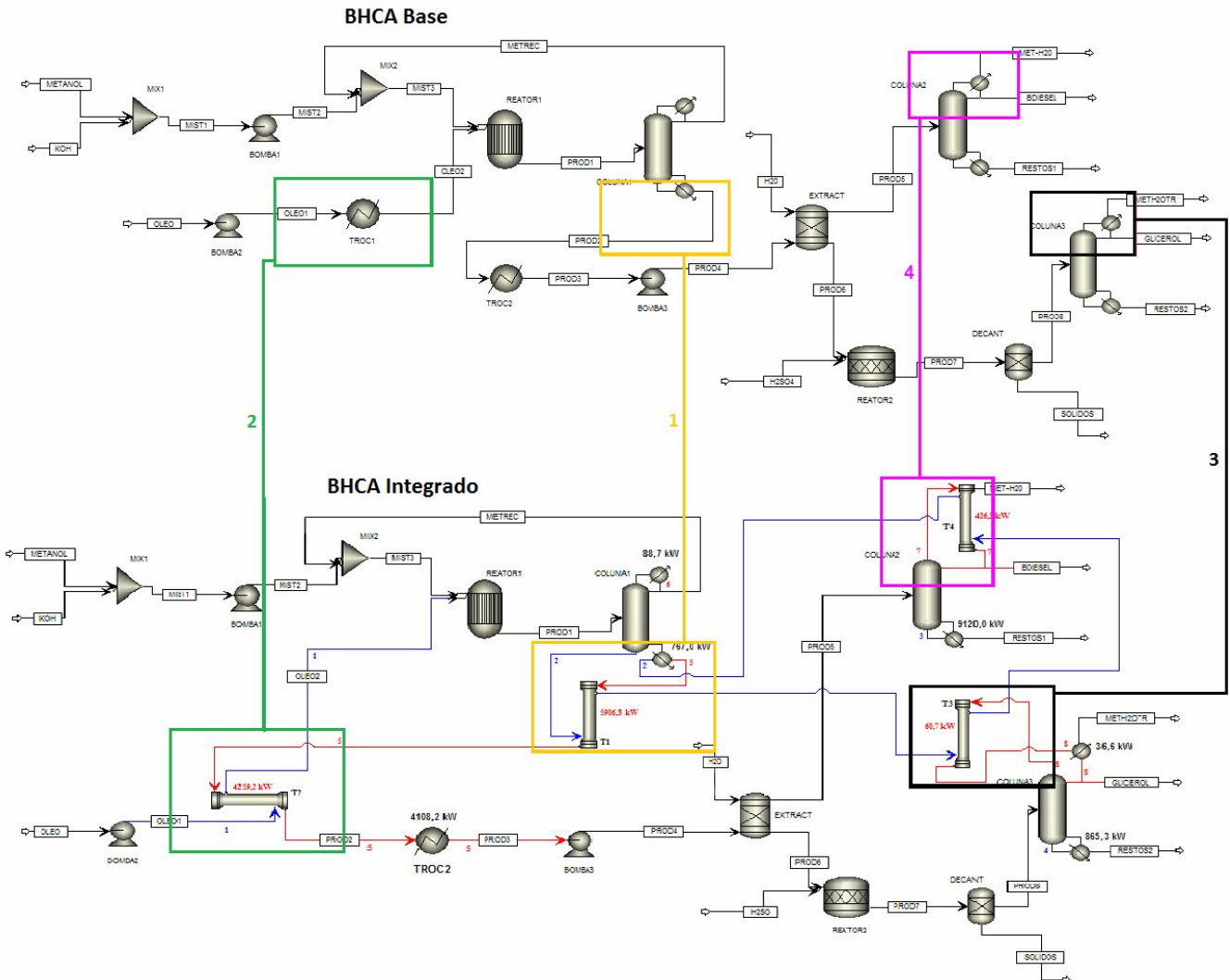
Figura 6.8 – Diferenças nos diagramas de processo BCHA base e BCHA integrado.
