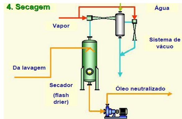
Figura 2.8 – Etapa da secagem do óleo bruto [30].
