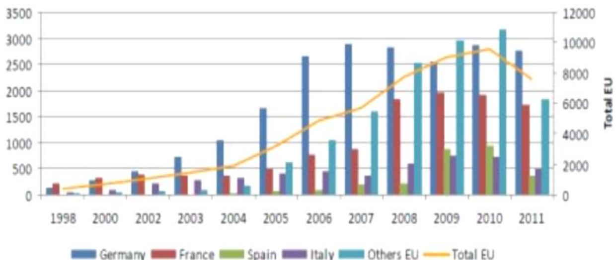
Figura 2.1 – Produção europeia registrada até 2010 e prevista para 2011 [27].
