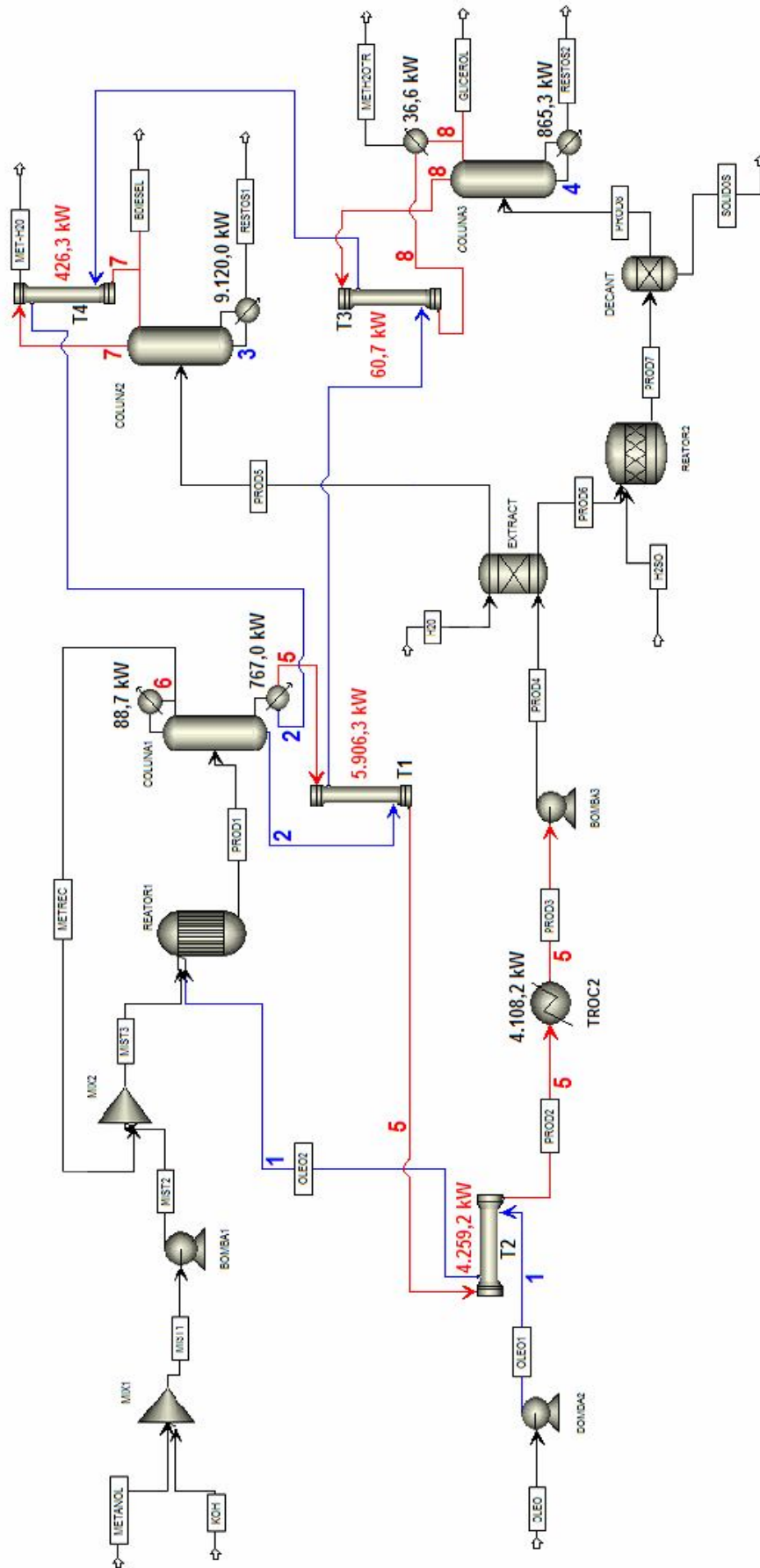
Figura 6.7 – Diagrama do processo BCHA após integração energética.
