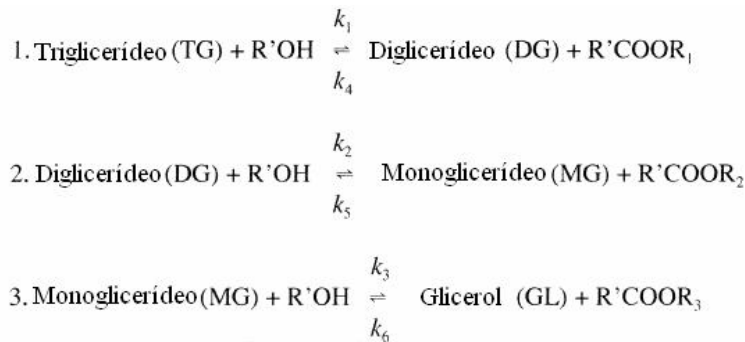
Figura 1.2 – Mecanismo da reação de transesterificação [17].
