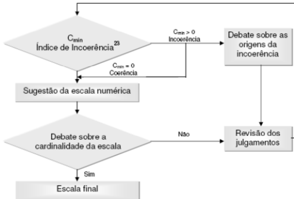
Figura 5 – Fluxograma geral do método MACBETH (Vilas Boas, 2006)
