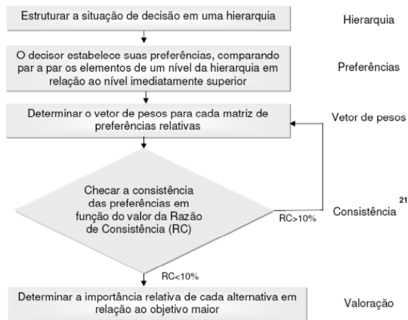
Figura 4 – Fluxograma geral do método AHP (Vilas Boas, 2006)
