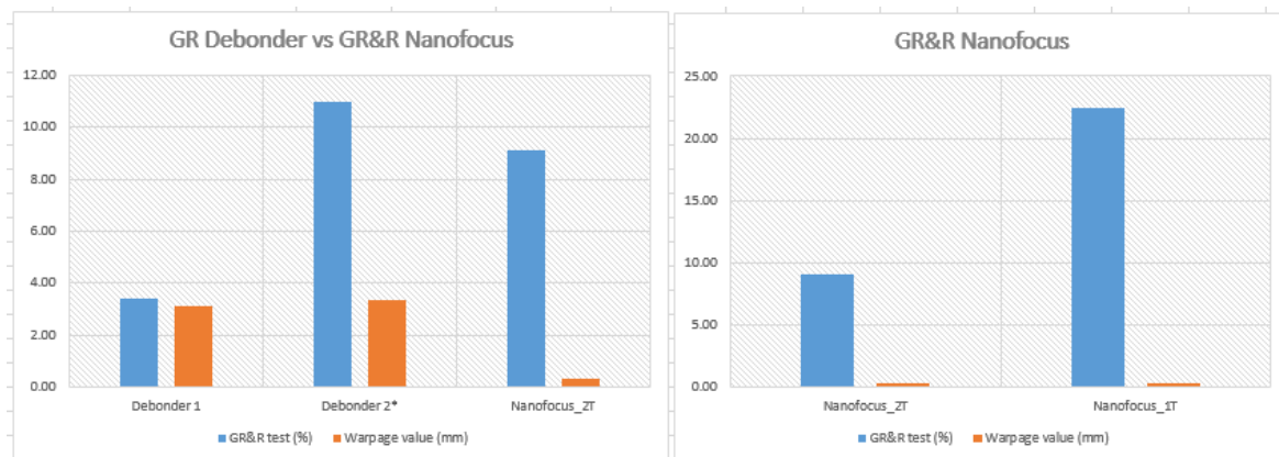
Figura 32 - Gráficos com os resultados do estudo GR e GR&R no processo de debond .
