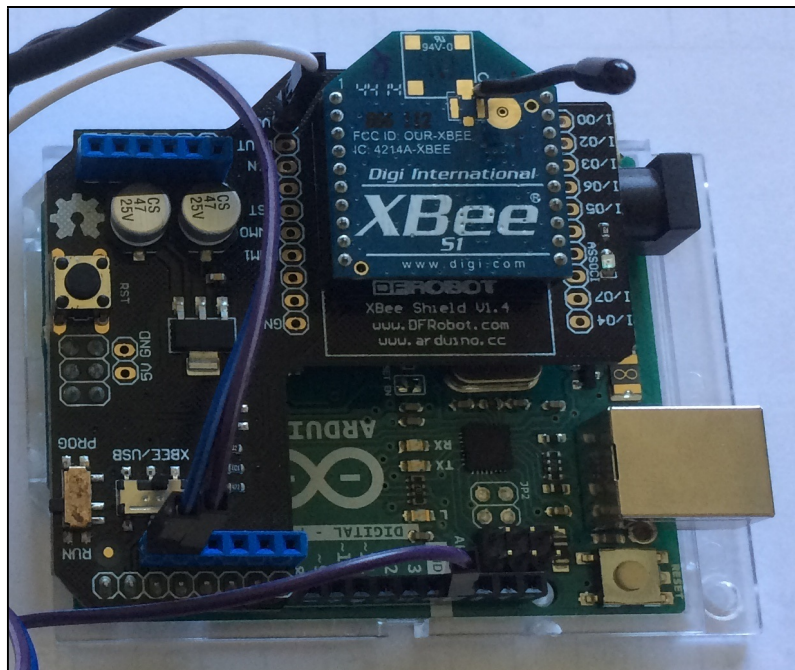
Figura 7 Arduino e placa ZigBee / XBee.
