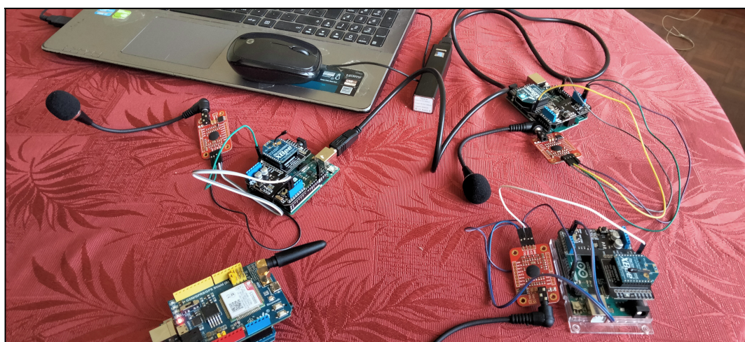
Figura 12 Foto dos três detetores de palavra e da central de controlo
