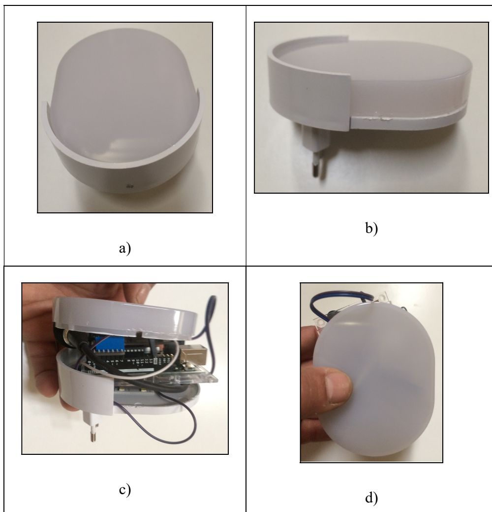
Figura 15 Detetor de palavra incorporado numa mini luz de presença.
