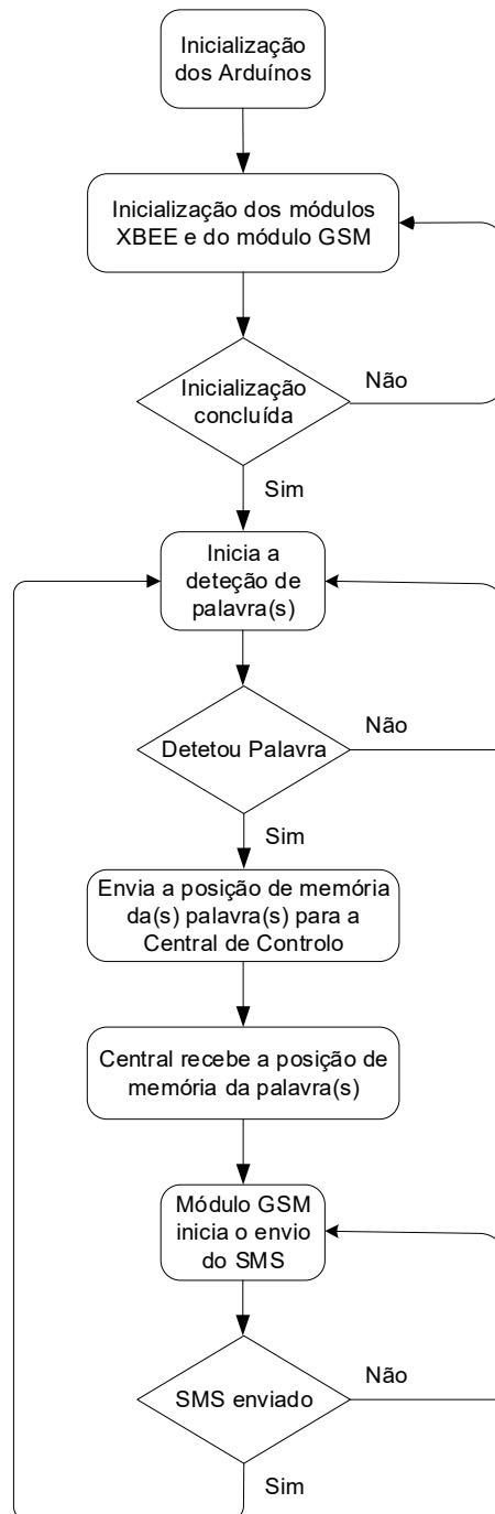
Figura 11 Fluxograma do algoritmo implementado no programa Arduino.
