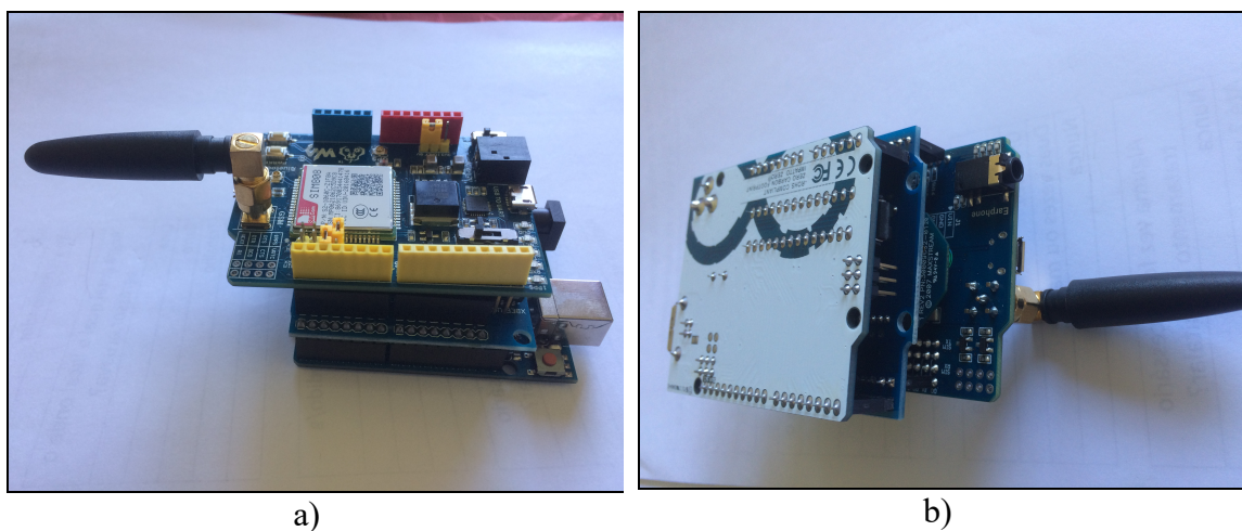
Figura 8 Interligação dos dispositivos da central de controlo. a) vista de cima e b) vista de baixo.
