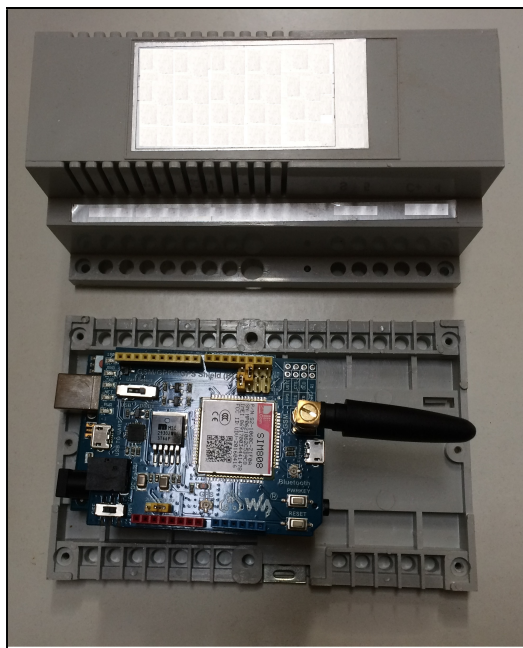
Figura 16 Invólucro com a central de controlo.
