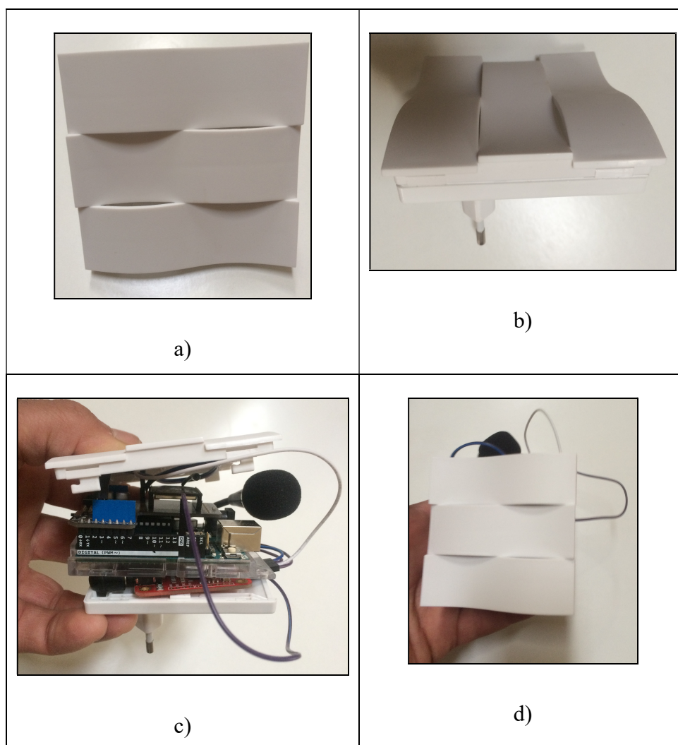
Figura 14 Detetor de palavra incorporado num ambientador
