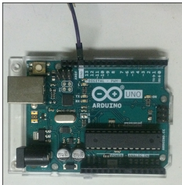
Figura 5 Arduino UNO R3.
