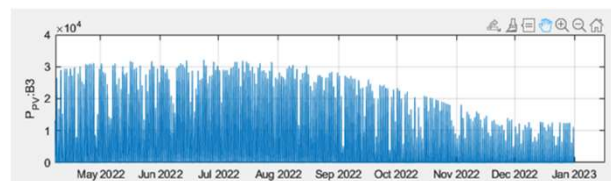
Figura 15. Potência solar durante o mês de dezembro
