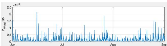
Figura 4. Potência eólica
