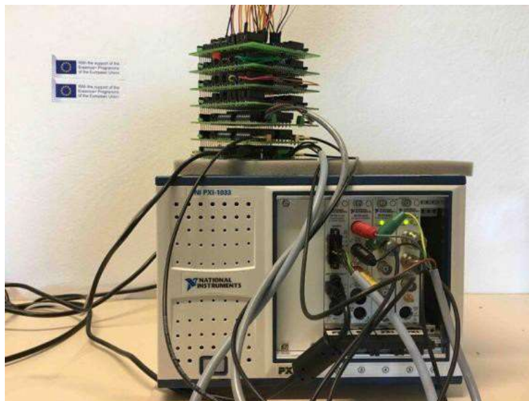
Figura 2. Equipamento instalado.
