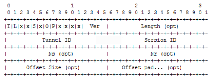
Figura 6 - Cabeçalho L2TP
