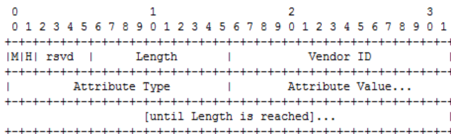
Figura 7 - Codificação AVP
