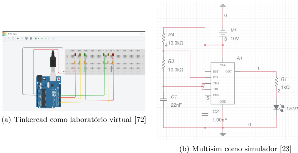
Figura 2.5: Laboratório virtual vs simulador
