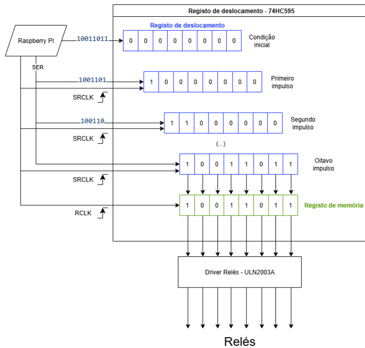
Figura 4.4: Envio de bits para o registro de deslocamento
