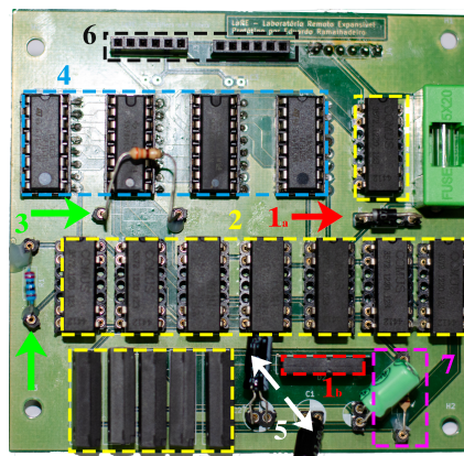
Figura 3.19: [Placa] rectificadores e filtros
