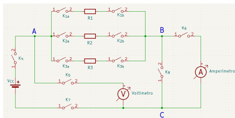
(a) Esquema implementado
