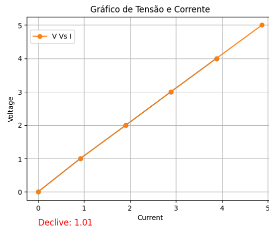
Figura 5.2: Gráfico da Lei de Ohm - 1 k \Omega - LaRE
