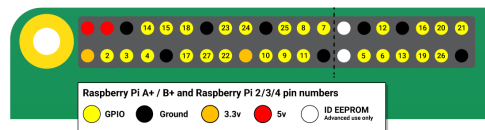
Figura 3.23: Representação alternativa dos GPIO [148]
