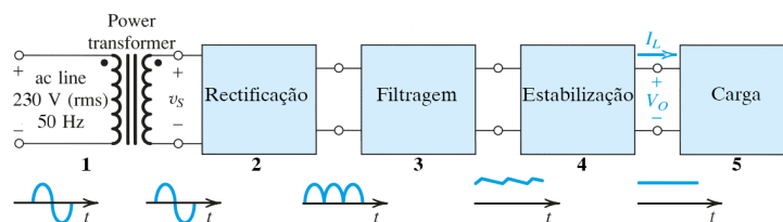
Figura 3.10: Diagrama de blocos da rectificação [144]
