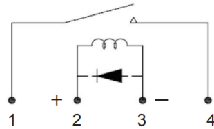
Figura 3.24: Esquema simplificado de um relé [150]
