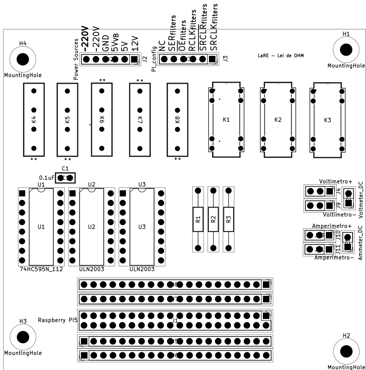
Figura 5: LaRE - Pinout [Lei de Ohm] Os símbolos ** indicam o pino 1 dos relés
