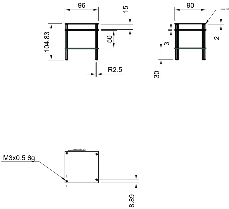
Figura 8: Dimensões mecânicas LaRE
