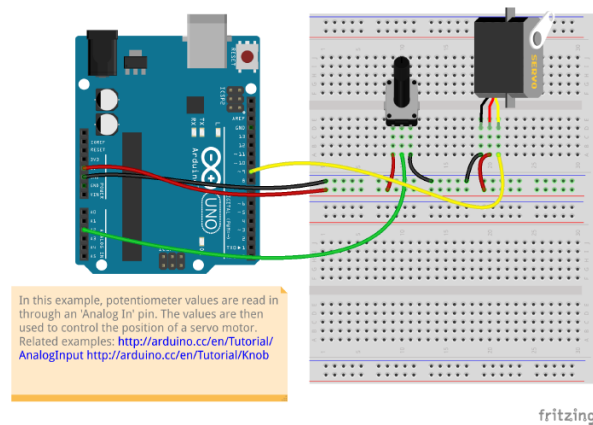
Figura 2.7: Laboratório virtual Fritzing exemplo
