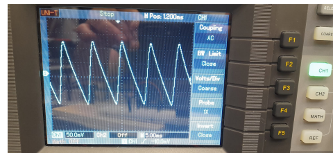
(b) Medição - B250C2300-1500
