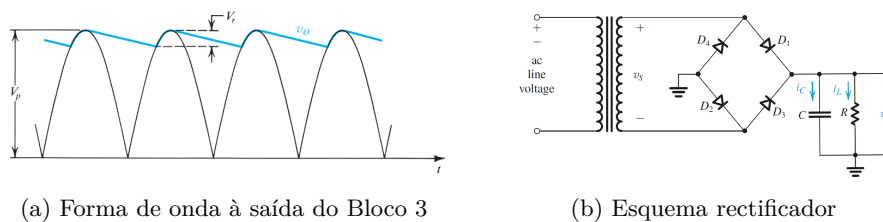
Figura 3.12: Rectificação onda completa [144]
