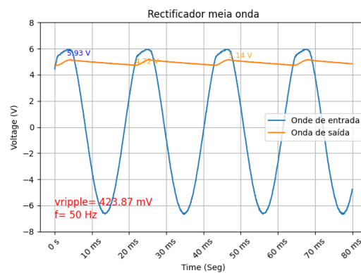
Figura 5.4: Tensão de ripple no LaRE - meia onda
