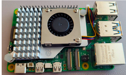
Figura 3.21: Raspberry PI5 com dissipador activo utilizado no LaRE
