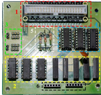
Figura 3.18: [Placa] Lei de Ohm
