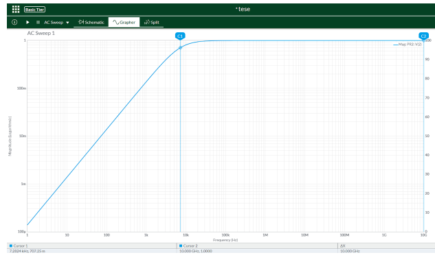
Figura 5.10: Frequência de corte - Multisim - Diagrama de Bode
