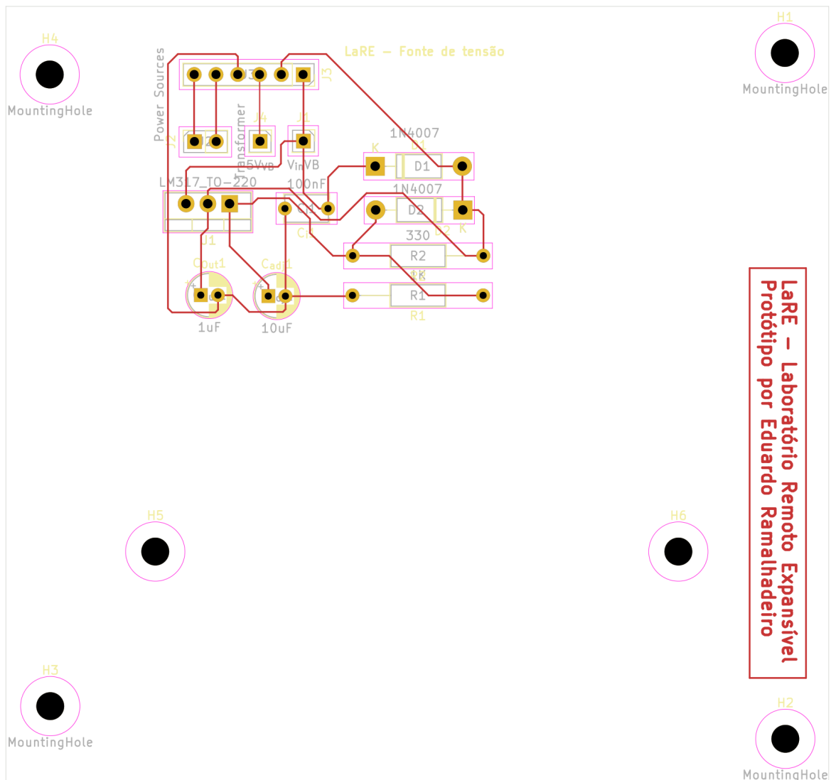
Figura 13: LaRE - PCB [Fonte de tensão]
