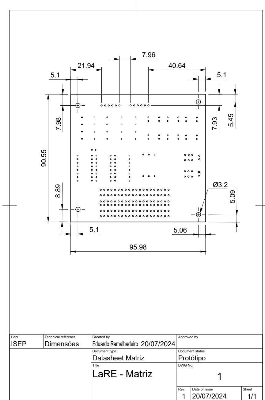
Figura 7: Dimensões mecânicas PC/104 - LaRE
