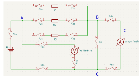
(b) Esquema com os relés duplos
