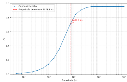
Figura 5.9: Frequência de corte - filtro passa-alto - Diagrama de Bode
