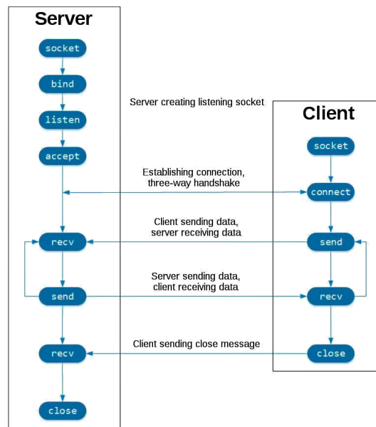
Figura 3.6: Fluxograma de uma chamada ao socket [142]
