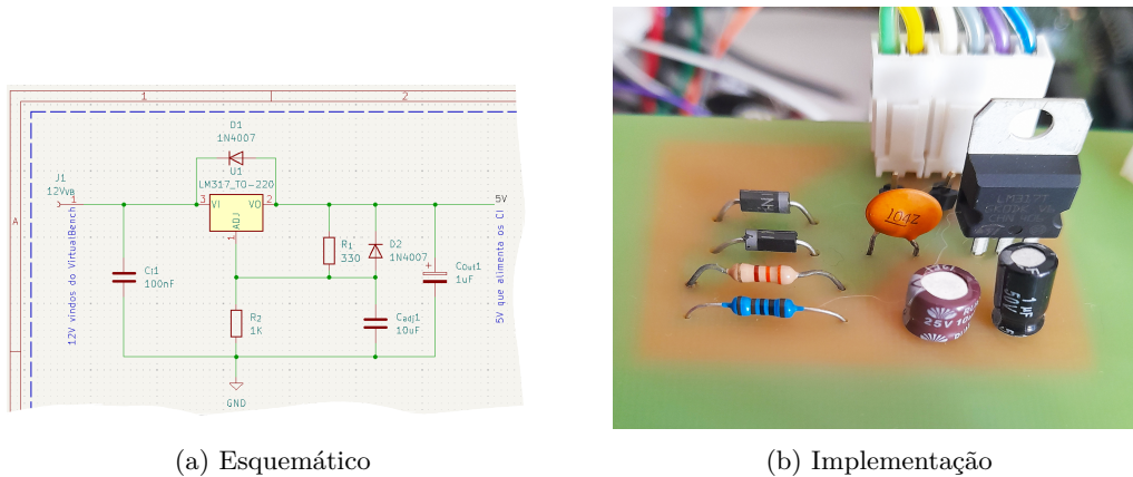
Figura 4.7: Fonte de 5 V [LM317]
