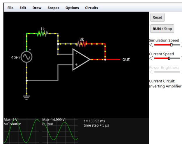
Figura 2.6: Simulador Falstad (exemplo) [24]
