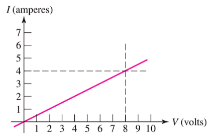
Figura 3.8: Gráfico da Lei de Ohm[143]
