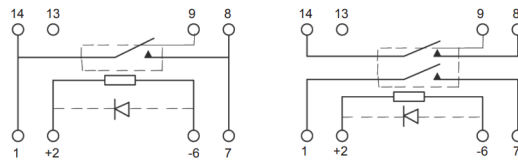
Figura 3.25: Relés SPST e DPST [150]
