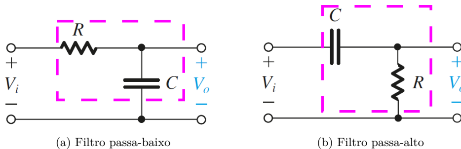
Figura 3.13: Esquemas dos filtros [144]
