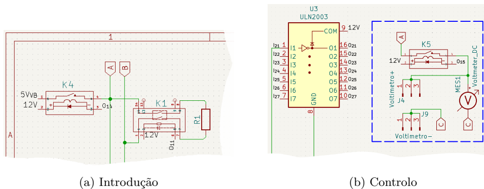
Figura 4.6: Implementação fontes de 6 V e 12 V
