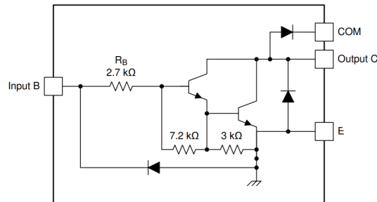
Figura 3.26: Diagrama de blocos ULN2003A [151]
