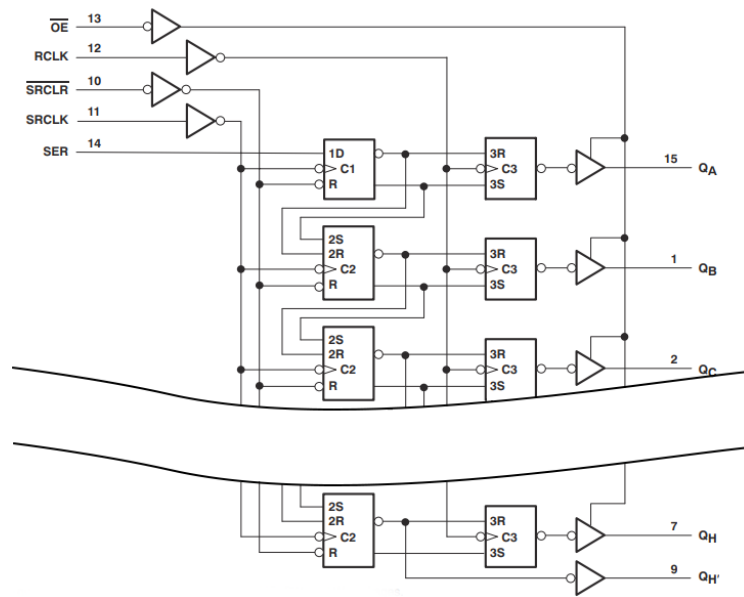
Figura 3.27: Diagrama [em corte] de blocos SN74HC595 [152]
