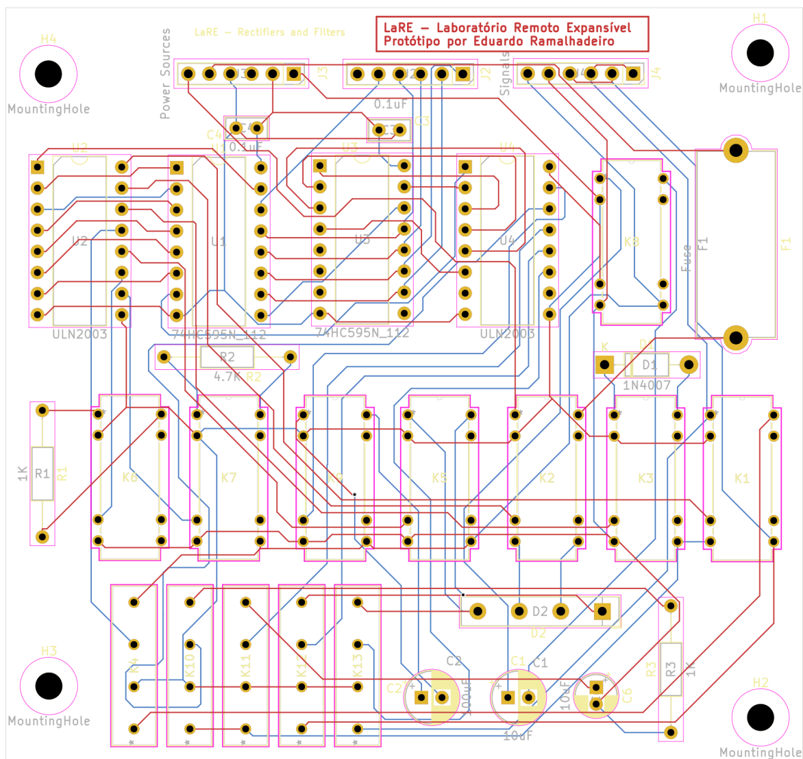
Figura 15: LaRE - PCB [Recfidores/Filtros]
