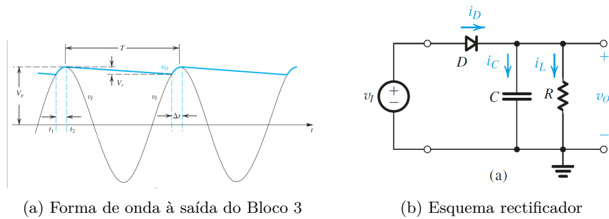
Figura 3.11: Rectificação meia onda [144]
