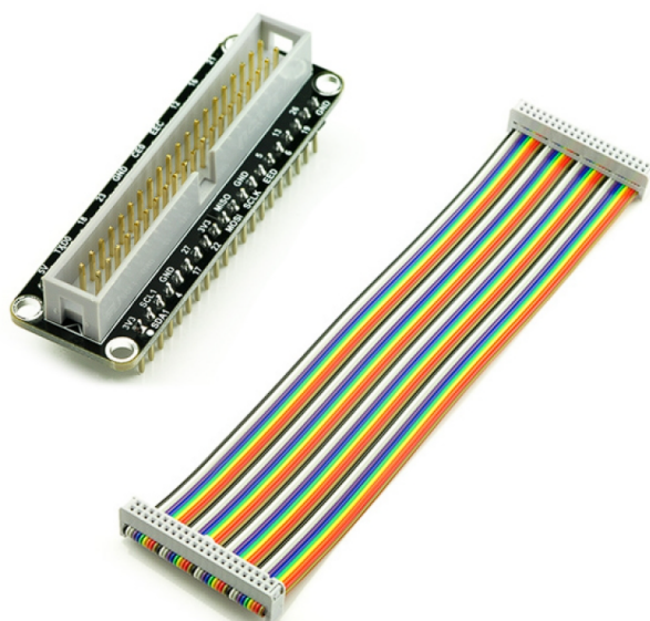
Figura 3: Ligação IDC 40 pinos [Macho/Fêmea]
