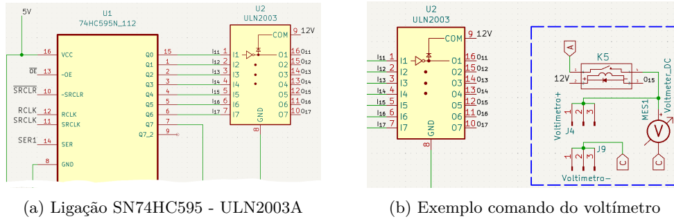
Figura 4.3: Exemplo de uso do SN74HC595 e ULN2003A
