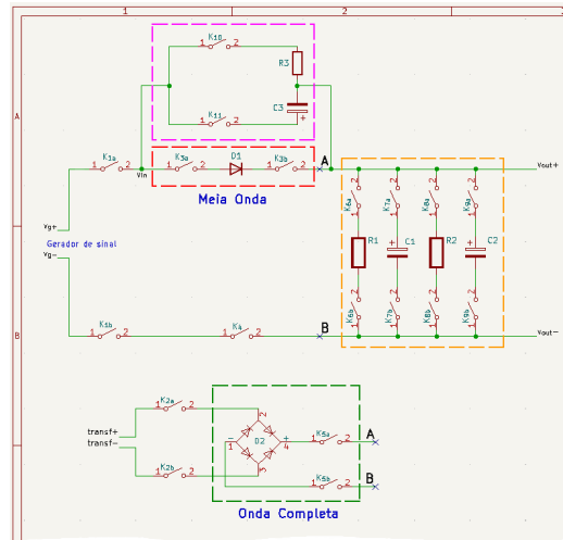
Figura 4.12: Esquema completo (simplificado) - rectificadores e filtros
