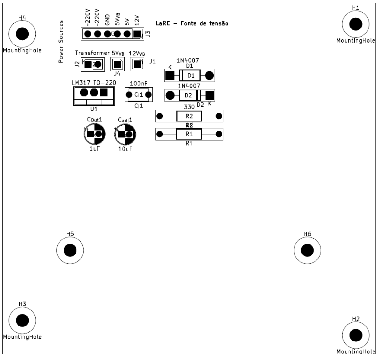
Figura 4: LaRE - Pinout [Fonte de tensão]
