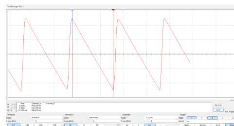
(b) Simulação Multisim
