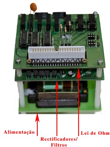
Figura 3.17: Matriz do LaRE
