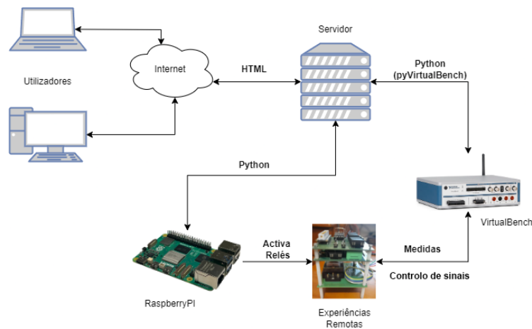
Figura 3.5: Arquitectura geral - LaRE
