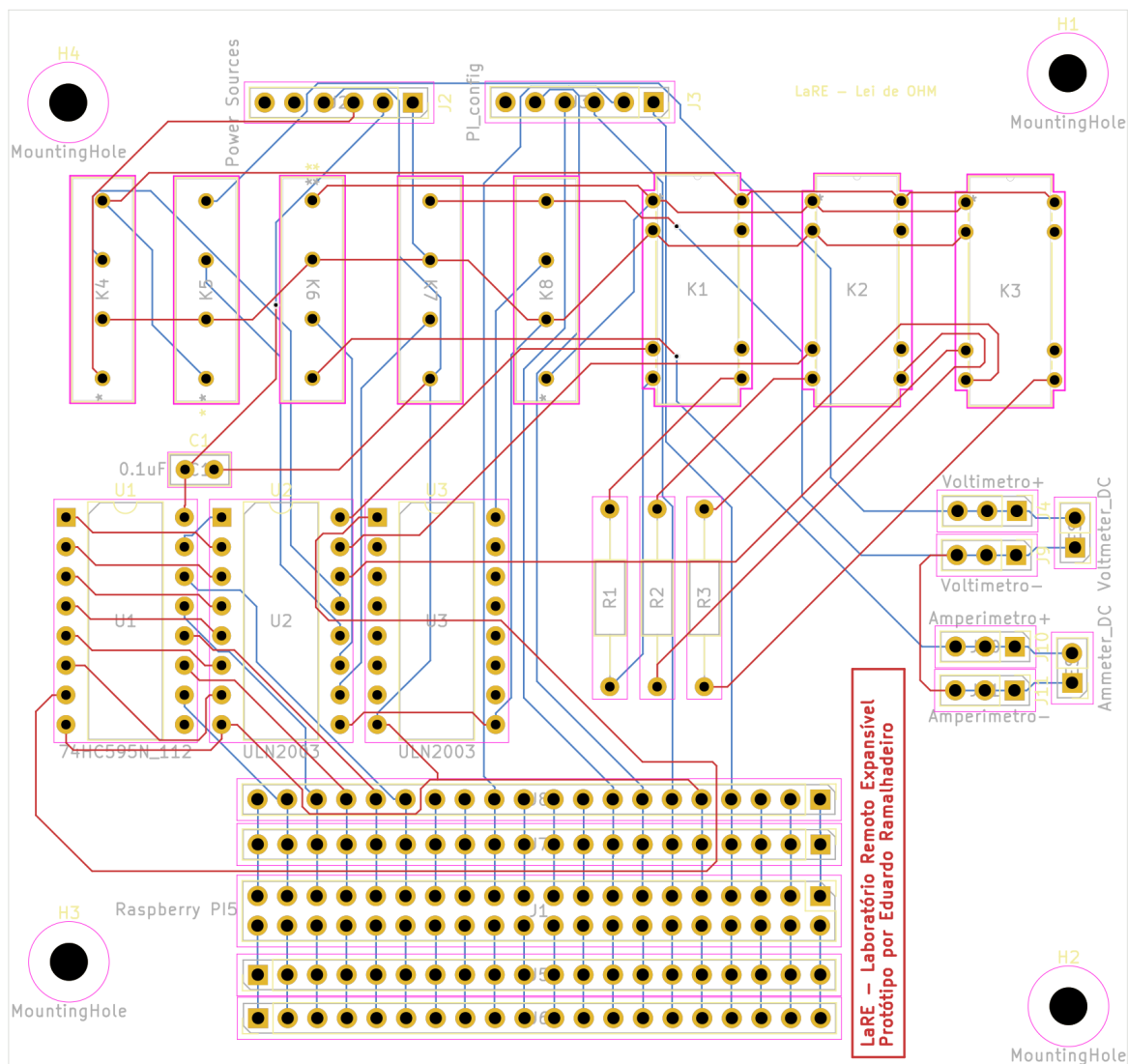
Figura 14: LaRE - PCB [Lei de Ohm]
