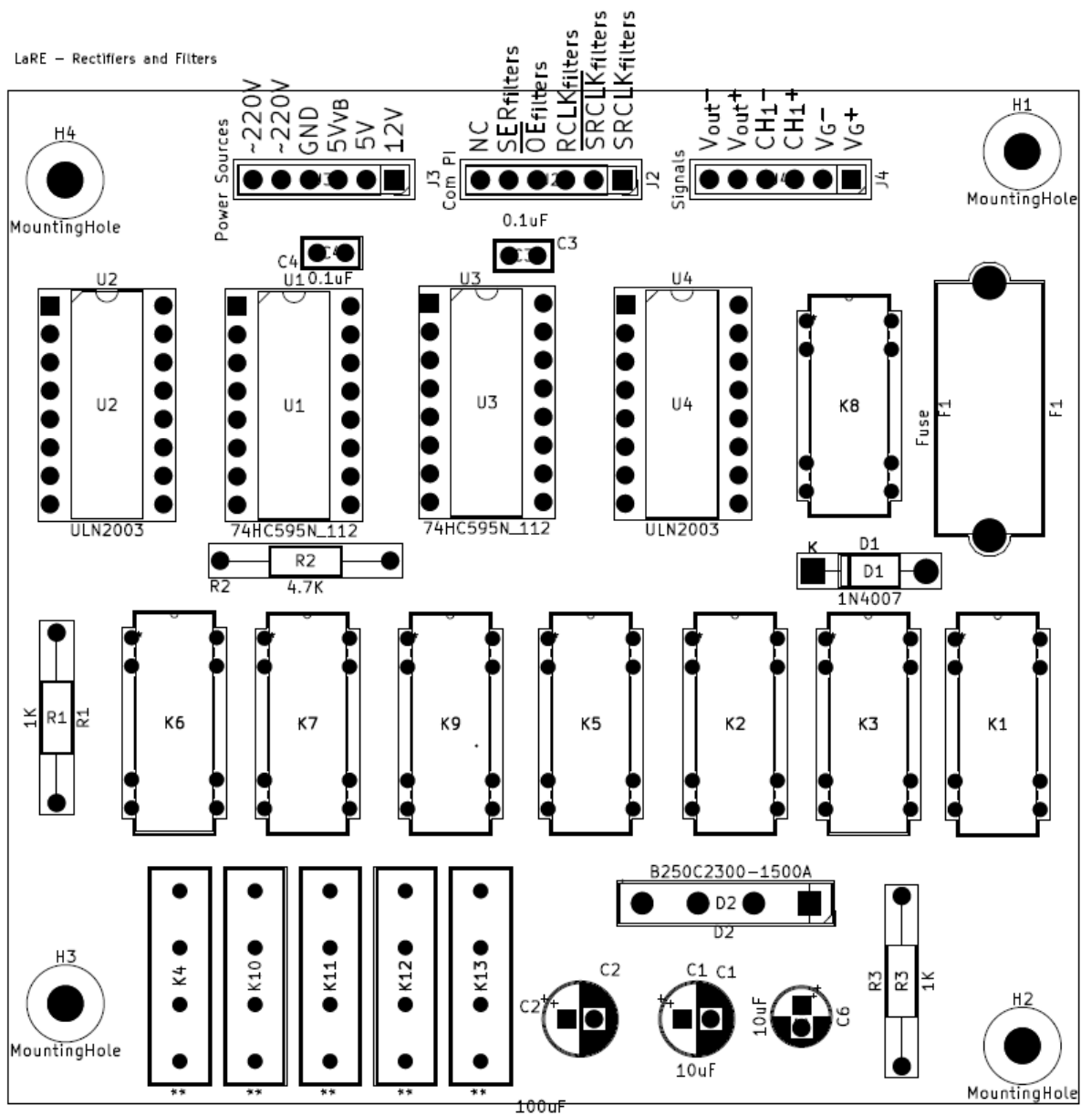
Figura 6: LaRE - Pinout [Rectificadores/Filtros]
