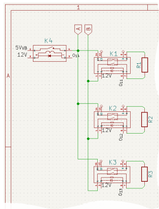
Figura 4.1: Exemplo de utilização de relés SPST e DPST
