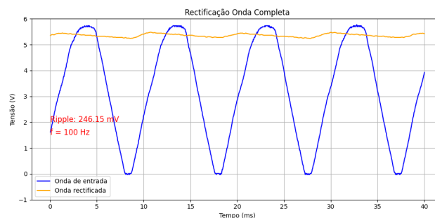
Figura 5.7: Tensão de ripple no LaRE - onda completa
