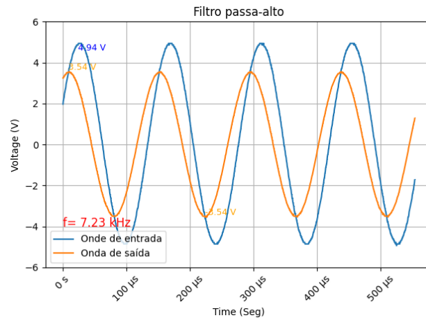
Figura 5.13: Frequência de corte - LaRE
