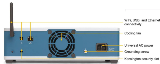
Figura 3.15: Painel traseiro VirtualBench VB-8012 [145].
