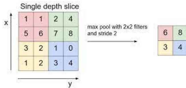
Figura 7 - Processo de max-pooling [24]
