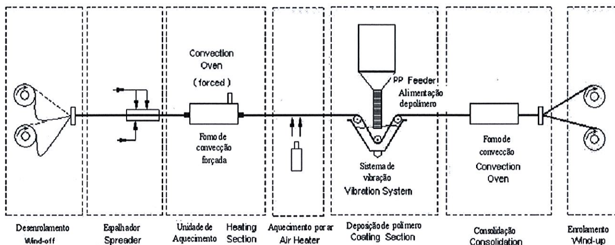
FP2 – Esquema da linha de deposição de polímero em pó. Powder coating line setup.
