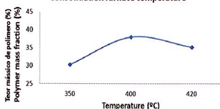
Temperatura do forno de consolidação Consolidation furnace temperature
