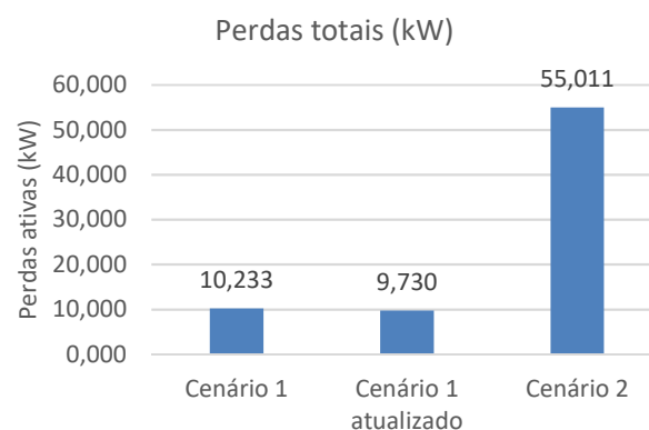
Fig.12 Comparação das perdas totais da rede nos diversos cenários
