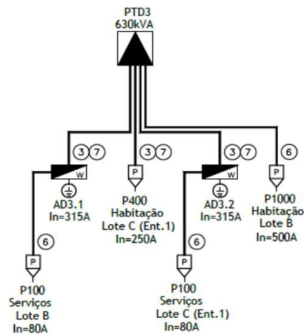
Fig.2 Esquema unifilar PTD3
