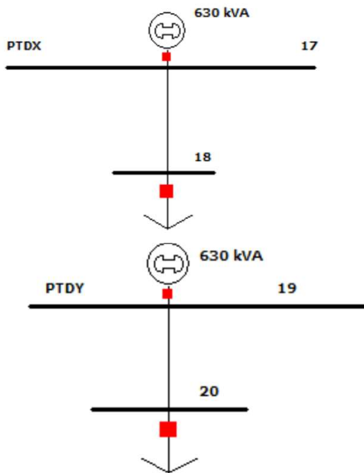
Fig.3 Esquema de rede do PTDX e PTDY em PowerWorld
