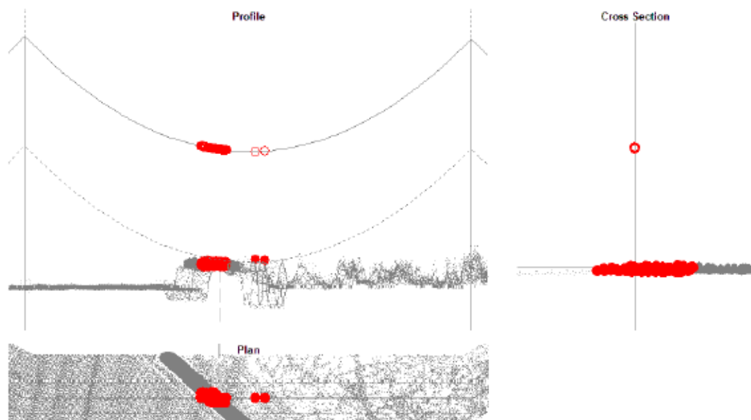
Figura 8. Exemplo de resultado PLS CADD de infração na distância à estrada
