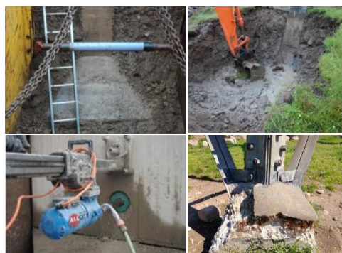
Figura 7. Recolha de provetes através de teste intrusivo
