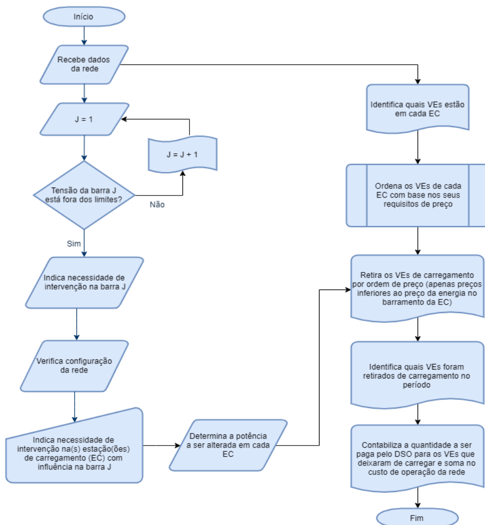
Figura 2. Fluxograma da Estratégia de carregamento dos VEs
