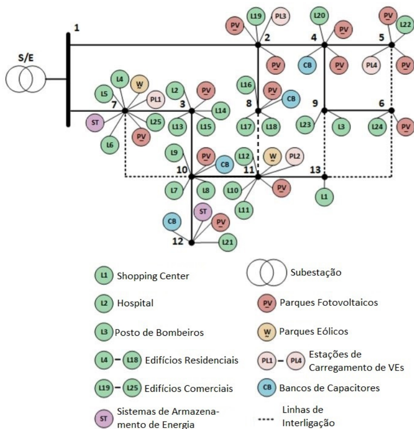
Figura 3. Diagrama Unifilar da Cidade Inteligente [10]
