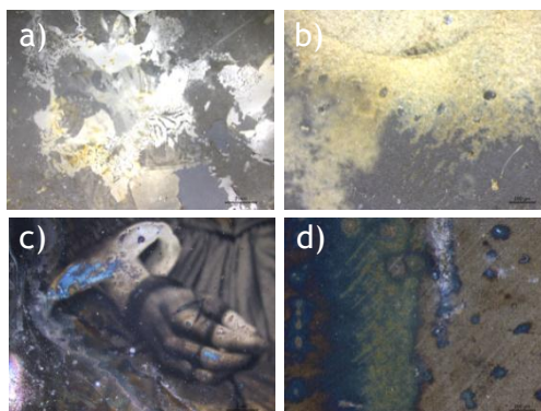
Figura 3: Imagens de microscopia ótica a diferentes ampliações 0.78x (a), c)) e 6.3x (b), d)) evidenciando a presença de diferentes patologias. a), b): negativo N1; c), d) :daguerreótipo D1.
